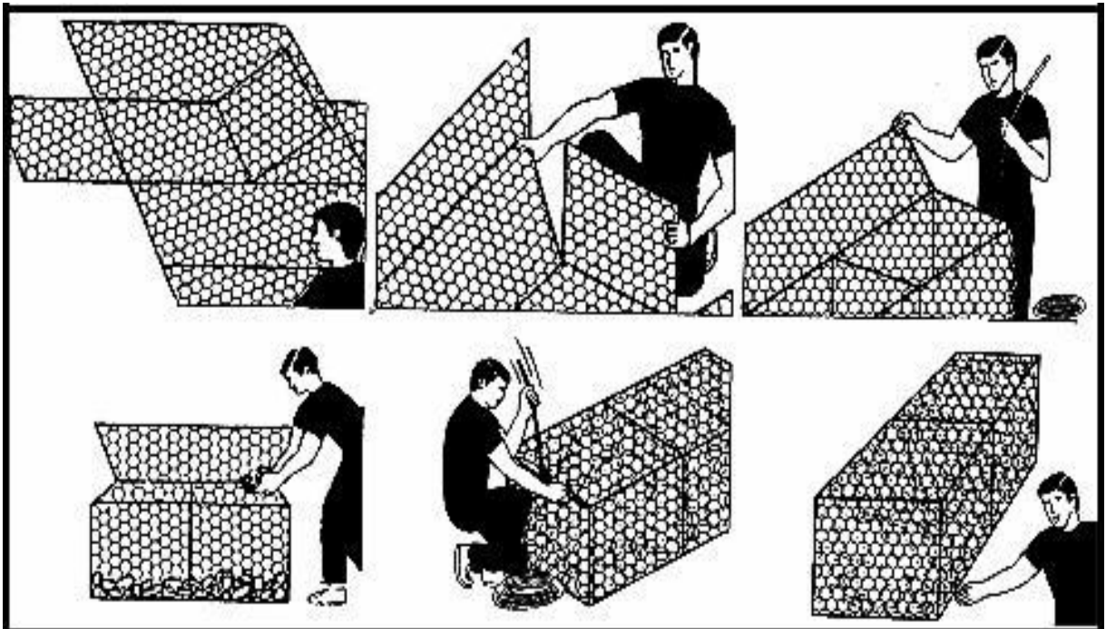
Figura 12. Pasos para el armado de las canastas de gavión
