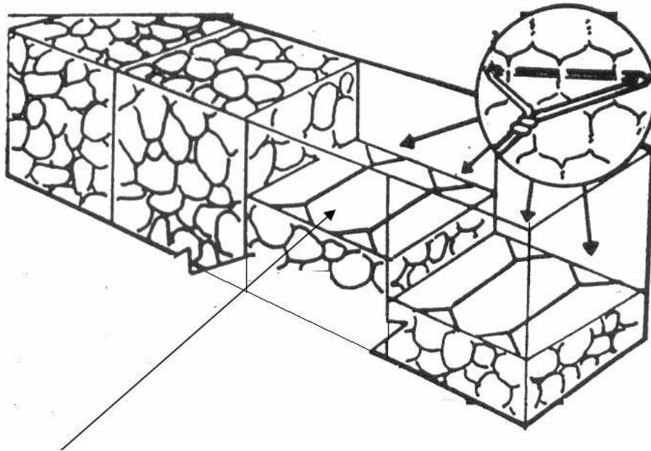
Figura 14. Amarre de tirantes en las cajas de gaviones
