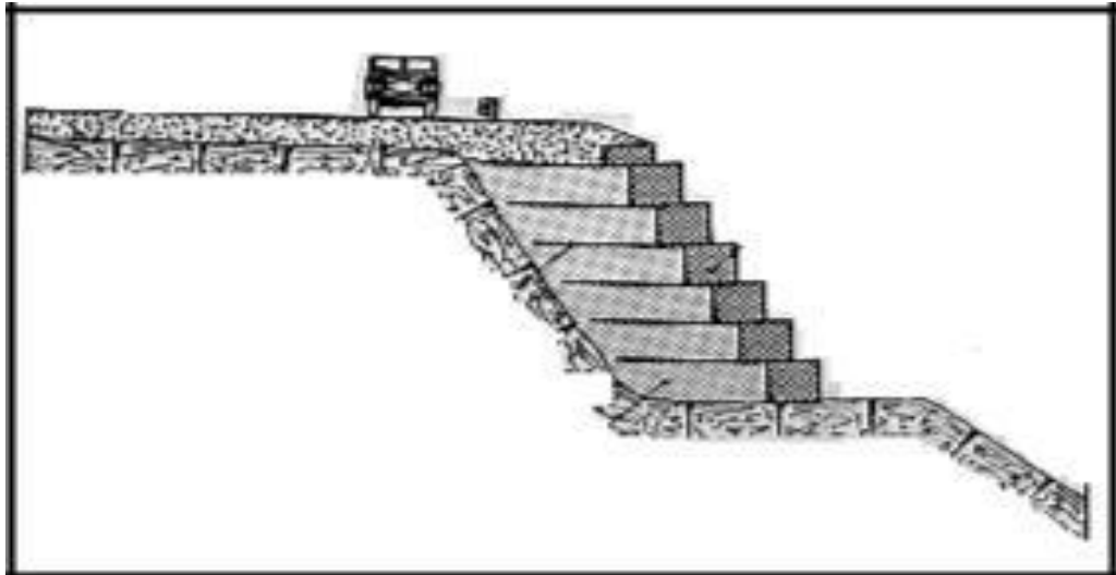
Figura 7. Protección de talud por medio de gaviones
